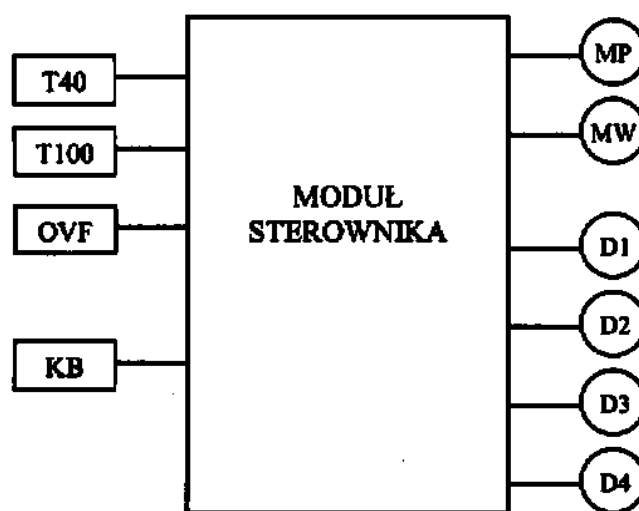
Rys. 1. Schemat blokowy nagrzewnicy na olej uniwersalny, typ WA 33.
