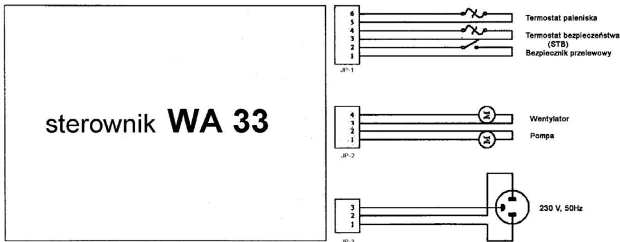
Rys.2. Sterownik pieca –wiązka przewodów
