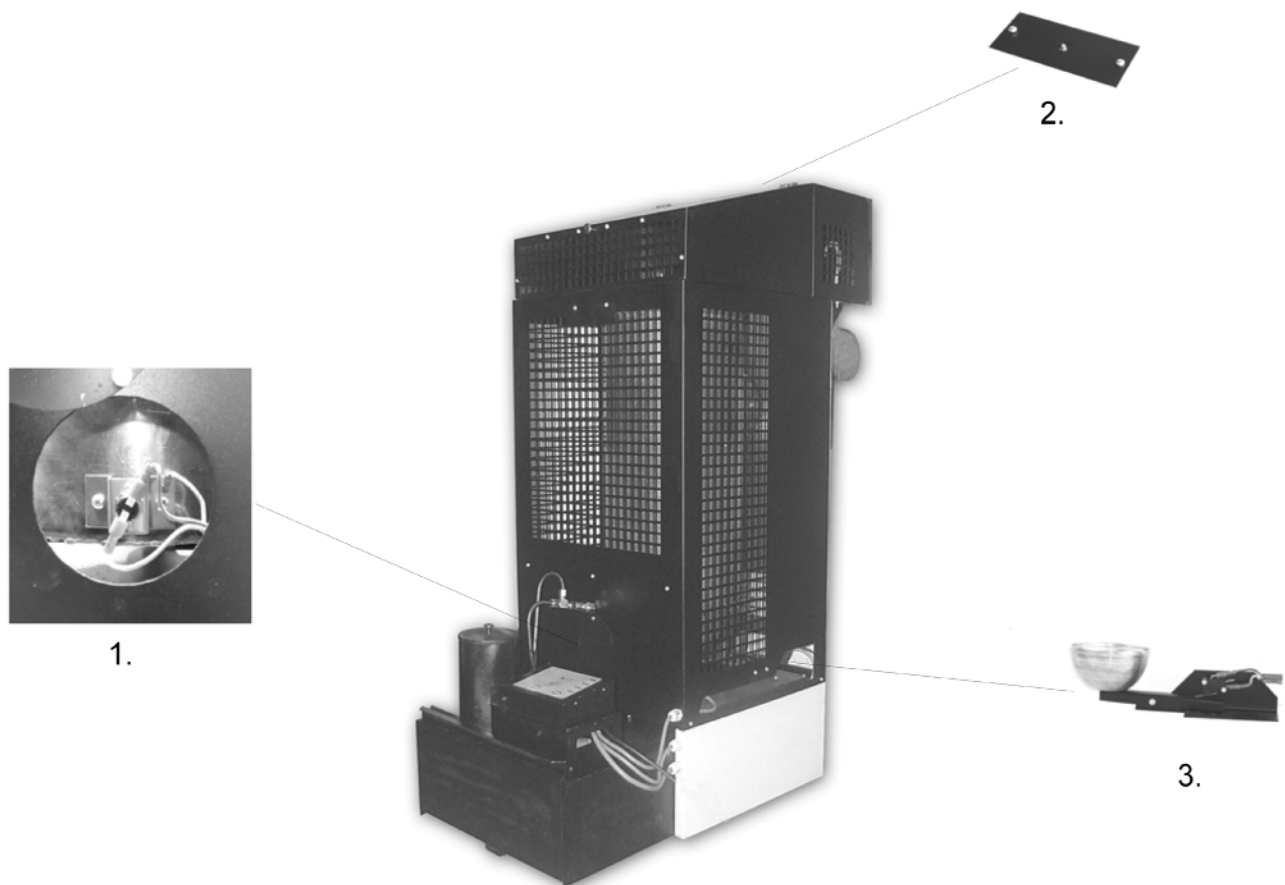
Rys.5. Rozmieszczenie elementów zabezpieczających nagrzewnicy:
