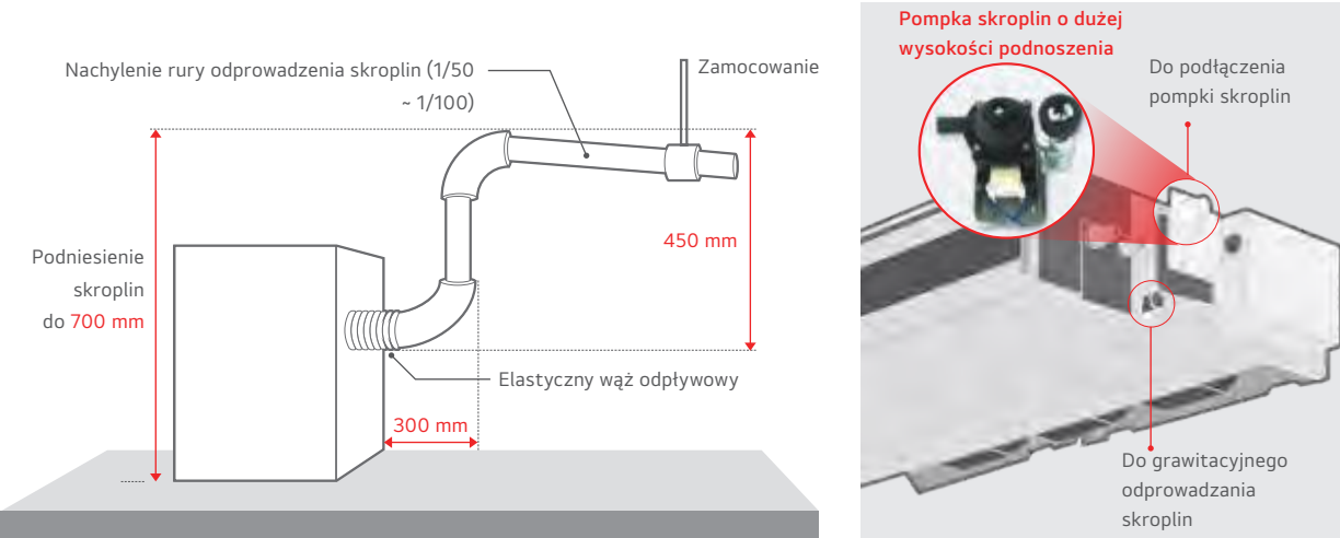
Standard Inverter: wyposażenie dodatkowe (ABDPG) / Kanałówki niskiego sprężu: wbudowane
