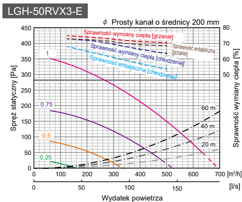
Krzywa charakterystyki
