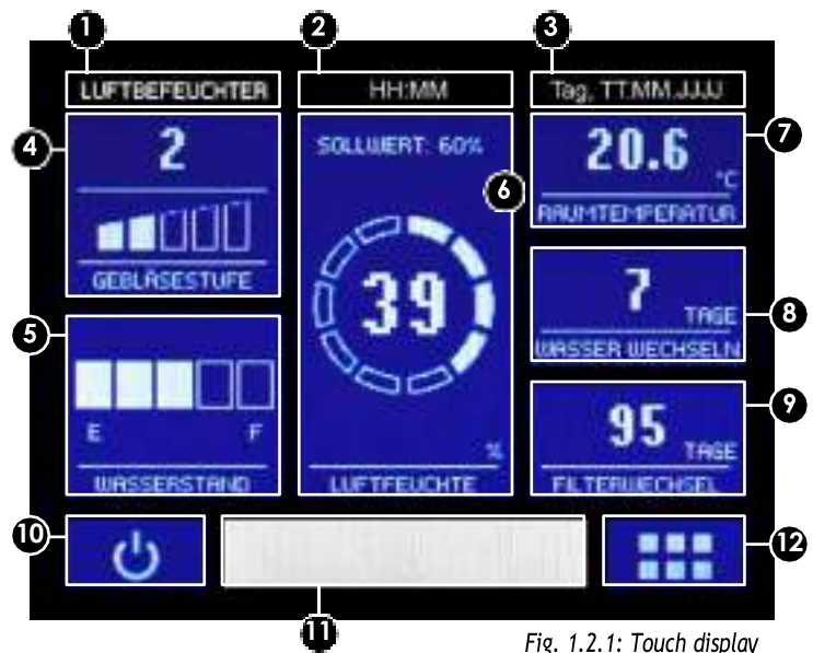
Fig. 1.2.1: Touch display
