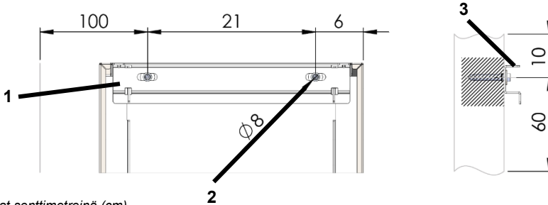
Kuva 5: Seinäkiinnityksen yleiskuva
