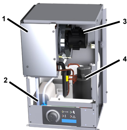
Fig. 3: Innvendige deler
