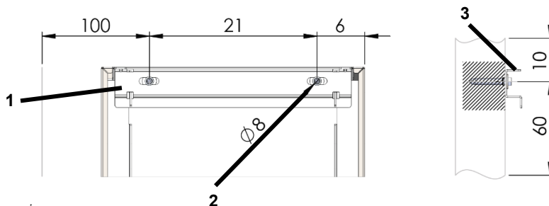
Fig. 5 : vue d'ensemble du montage mural
