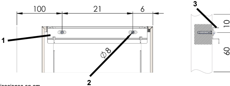
Fig 5: Descripción del montaje en la pared
