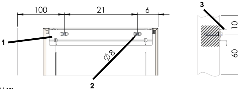
Fig 5: Oversikt veggfeste
