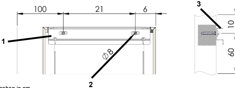
Fig 5: Übersicht Wandbefestigung
