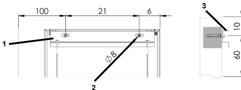
Rys. 5: Przegląd mocowania ściennego
